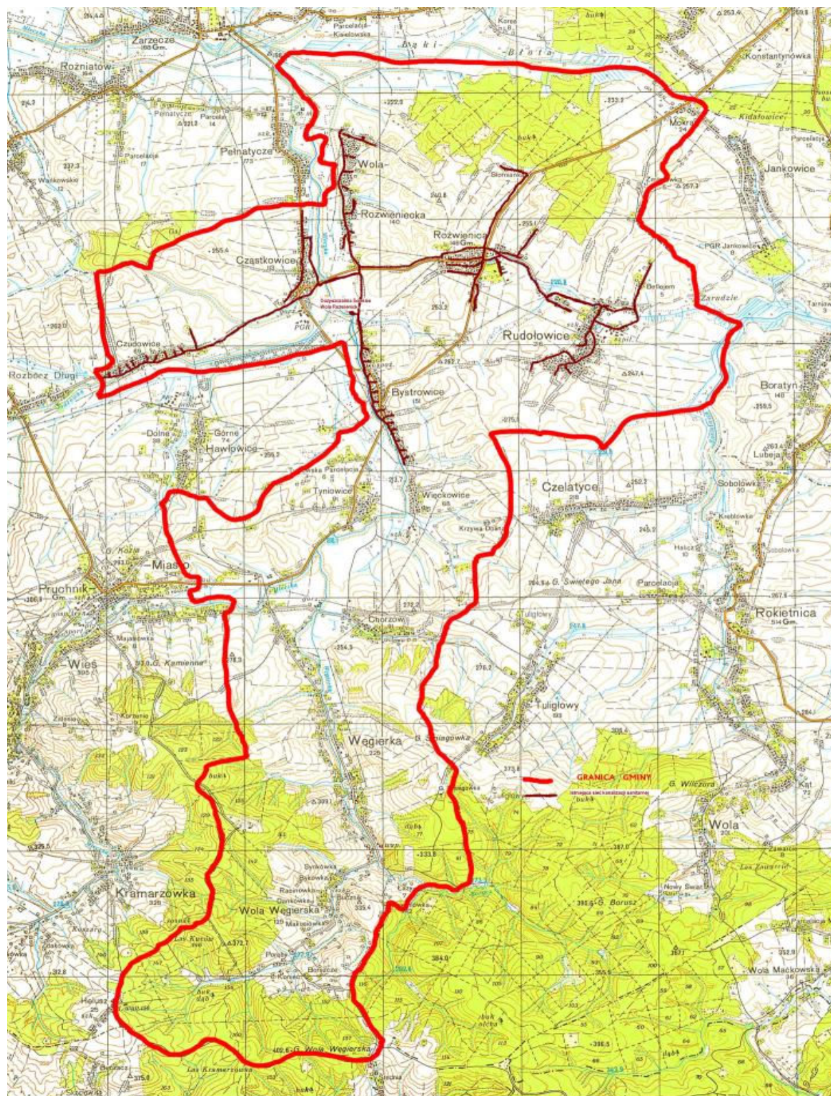
Rys. Nr 3 Sieć kanalizacyjna gminy Roźwienica.
