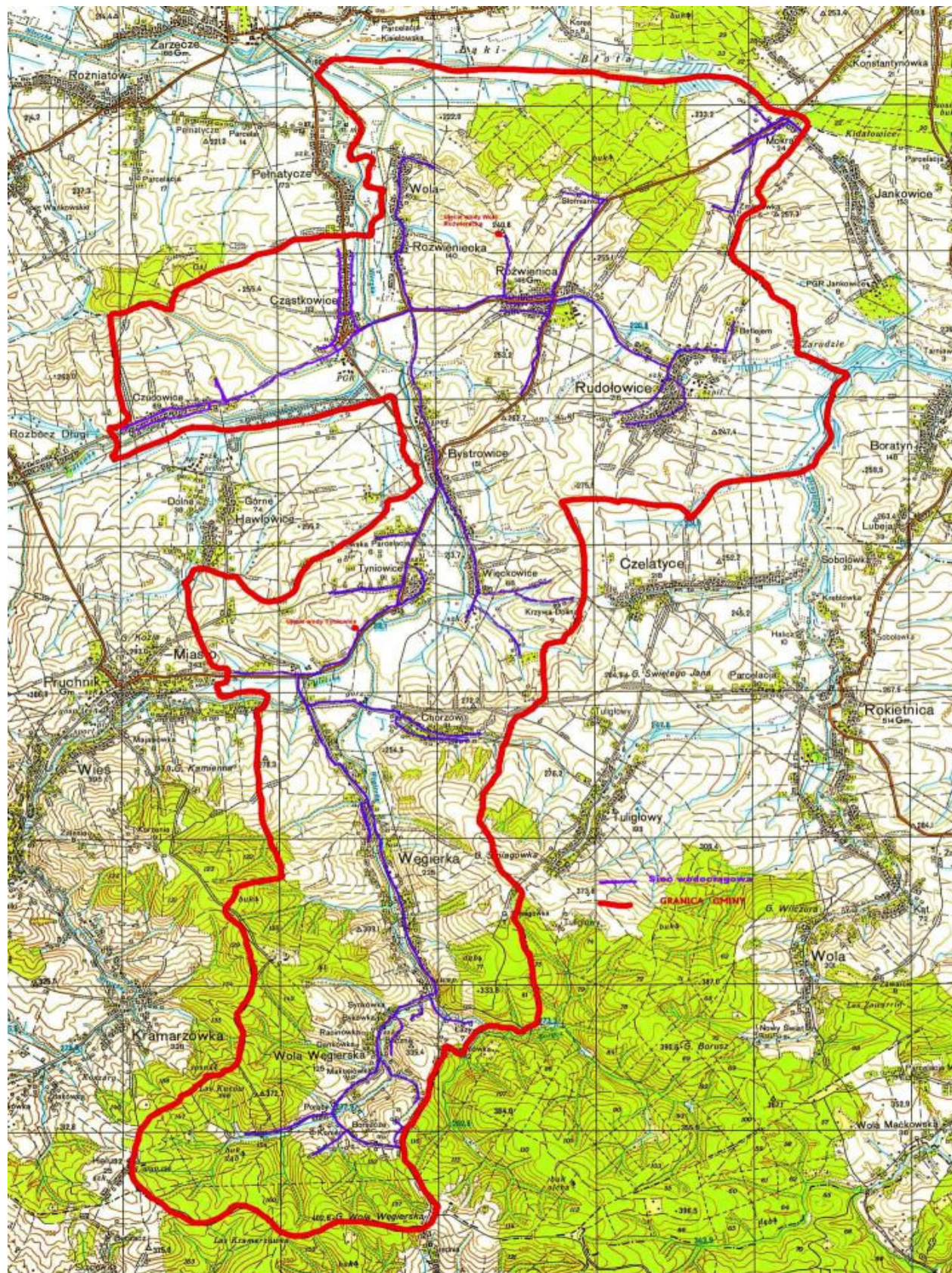
Rys.Nr 4 Zwodociągowanie gminy Roźwienica
